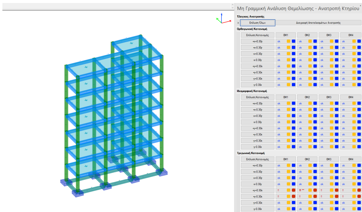
Εικόνα Σφάλμα! Δεν υπάρχει κείμενο καθορισμένου στυλ στο έγγραφο. -11: Αποτελέσματα μη γραμμικής ανάλυσης όλων των κατανομών φόρτισης.
