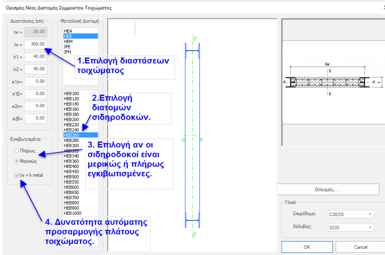
Εικόνα 1 – Διάλογος εισαγωγής διατομής σύμμεικτου υποστυλώματος.
